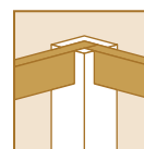
Vigas de 8x20 cm.
